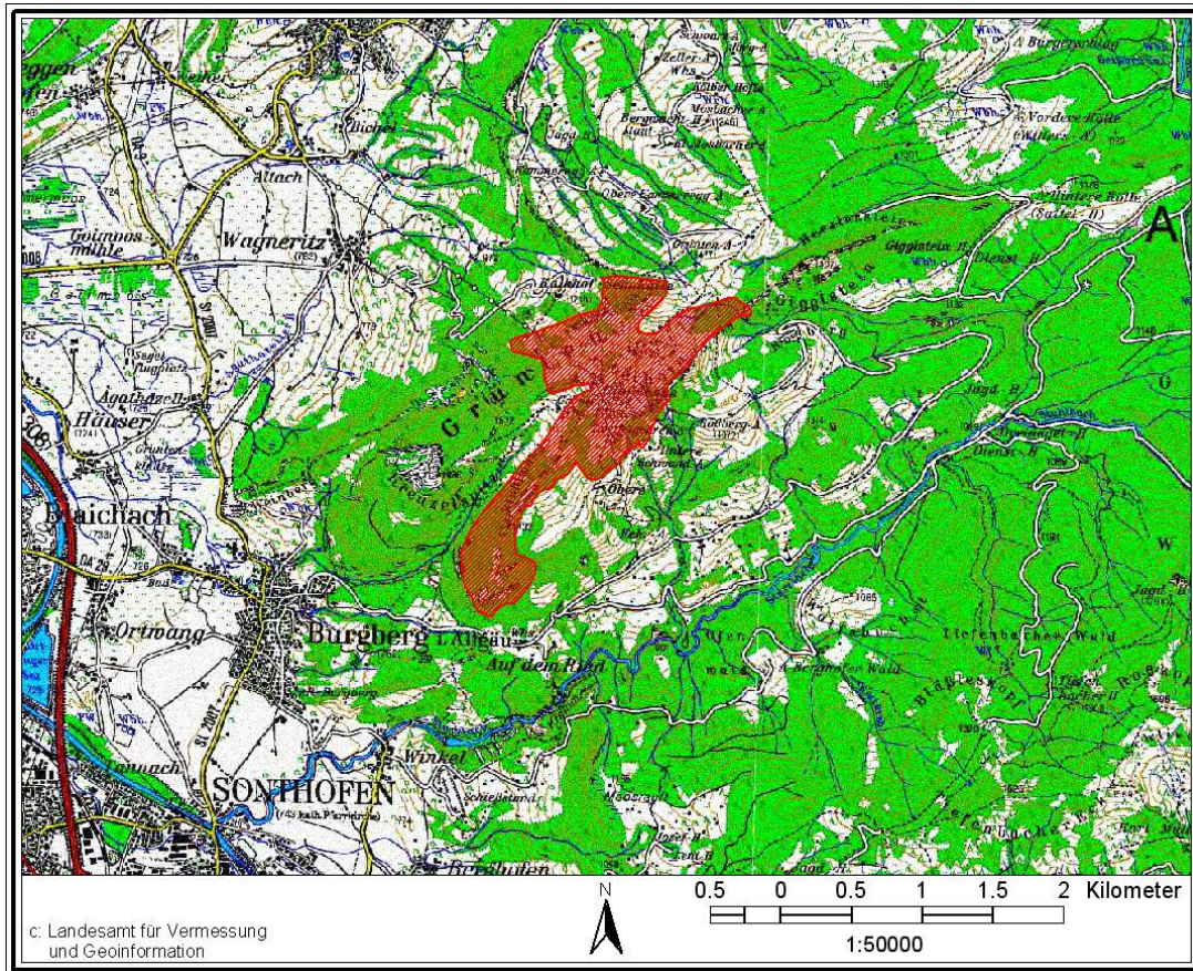
Abb. 3 : Übersichtskarte zur Lage des Gebietes
