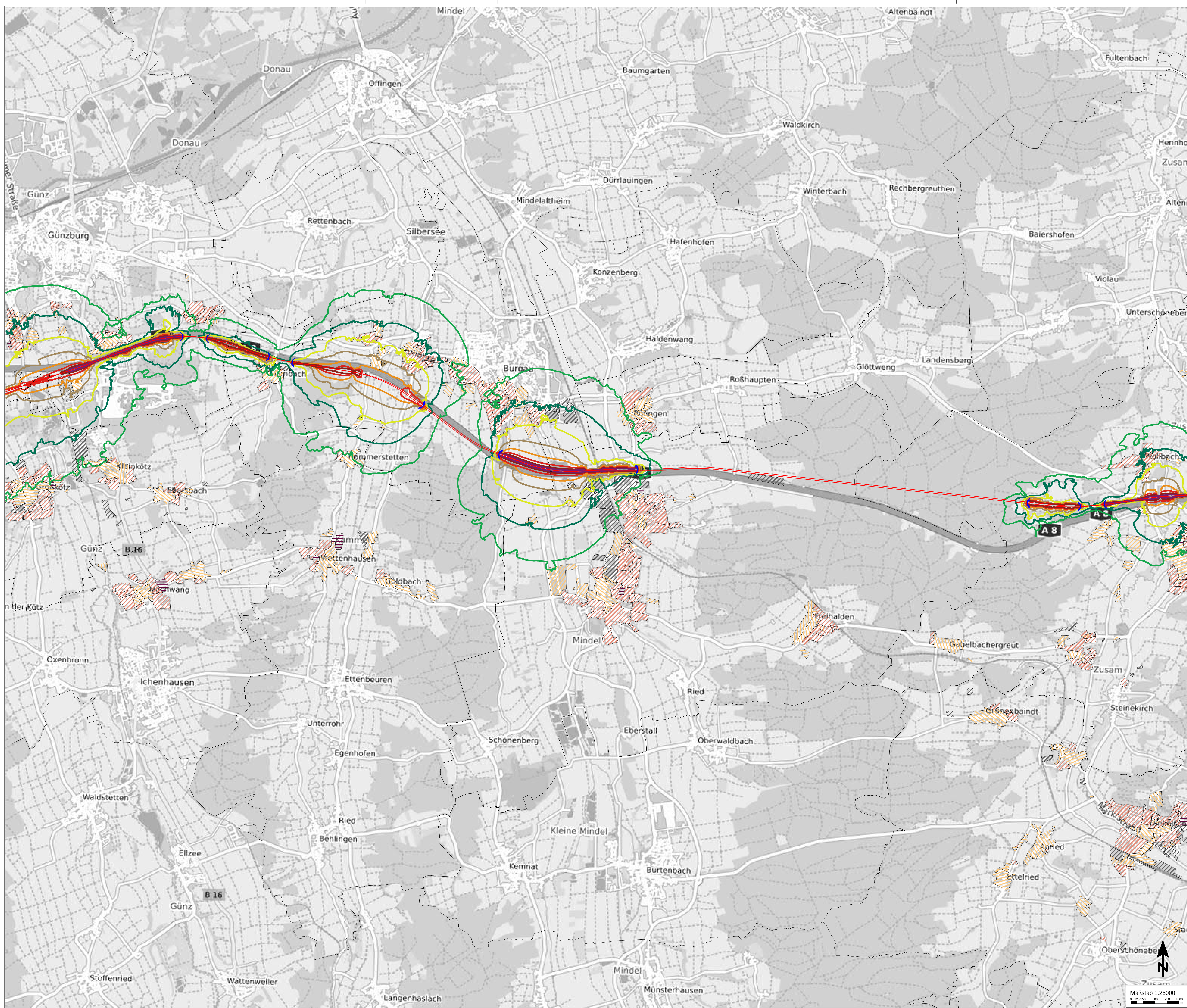
Isophonenkarte Raumordnungsverfahren NBS/ABS Ulm-Augsburg Variante Orange Tiefbahnhof Zusamtal, Beurteilungspegel Nacht Anlage_Orange Tiefbahnhof Zusamtal_2_2
